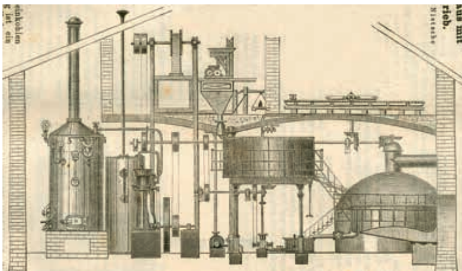
Obr. 2 Typizovaná varna Raimunda Nietscheho z roku 1876, kterou můžeme předpokládat i v Lukavci. Zleva stojatý parní kotel a malý parní stroj, který pohání hlavní transmisi varny, dále vystřávací a zároveň scezovací otevřená kád', nad kterou je umístěný šrotovník a vpravo kotel na přímý otop, nad varnou je umístěn chladicí štok s větrákem (Anonym, 1876).
