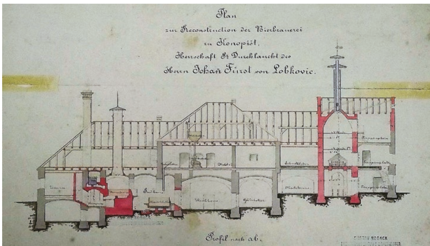
Obr. 1 Plán přestavby pivovaru na Konopišti z roku 1868 od firmy Noback & Fritze. Zdroj: SOA Praha, Velkostatek Konopiště, dodatek – Mapy, plány a nákrty, číslo plánu 93. (výřez)
