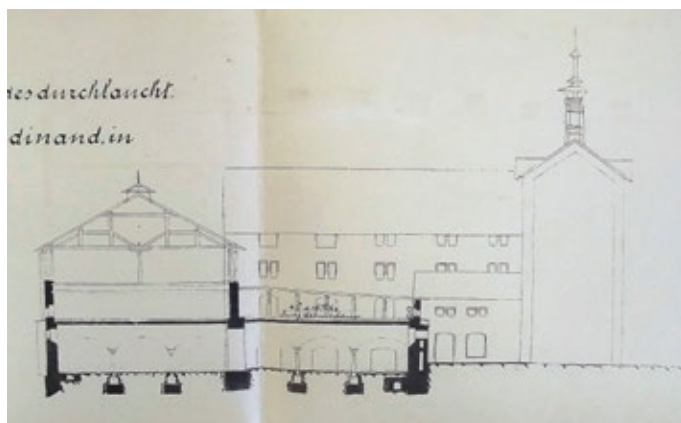
Obr. 3 Plán elektrifikace sladovny firmou Siemens & Halske z roku 1897 se zobrazením párníku chladicích stoků. Zdroj: SOA Praha, Ústřední ředitelství, inv. č. 64, signatura LIV/1, kart. č. 20. (výřez)
