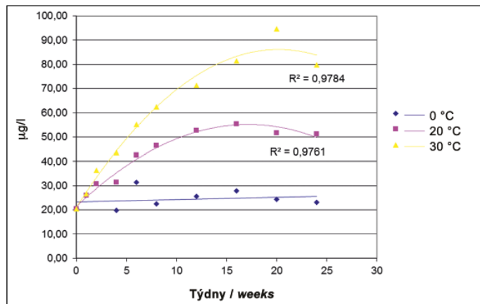
Obr. 3e Závislost obsahu vybraných sloučenin na délce staření – Fenylnacetaldehyd / Fig. 3e Dependence of the concentration of selected substances on the length of aging – Fenylnacetaldehyd
